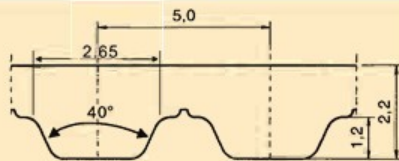
TIP T 5 - HATVE 5 mm
