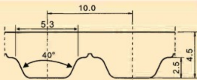
TİP T 10 - HATVE 10 mm
